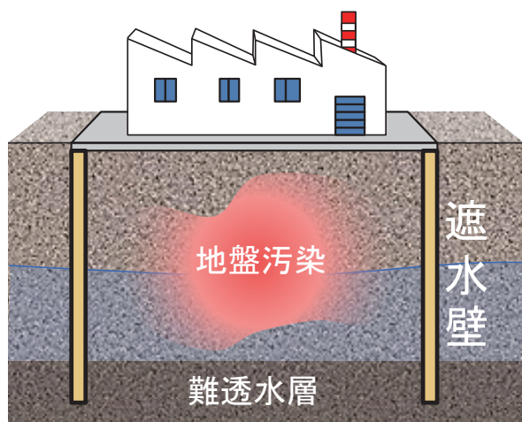
図-1 遮水壁による地盤汚染の封じ込め
