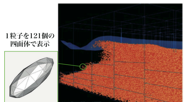
図-6 流れの中の100万個の粒子群運動の計算例
