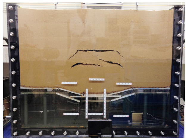
図-4 不同沈下時発生時のジオシンセティッククレイライナーの挙動を解析するための模型実験状況
