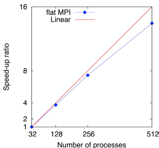
図-3 衝撃波の計算の並列化効率
