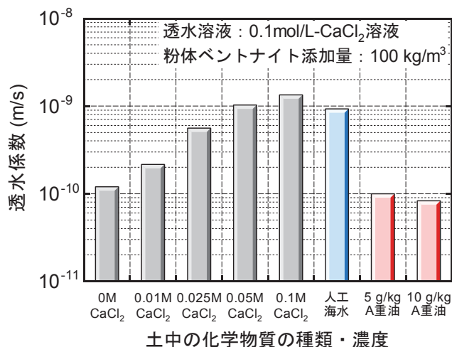
図-2 土中の化学物質とソイルベントナイトの遮水性
