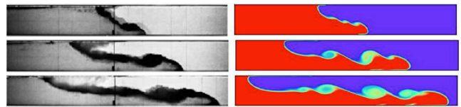
図-4 lock-exchange問題の実験 (Lowe, 2005) と計算
