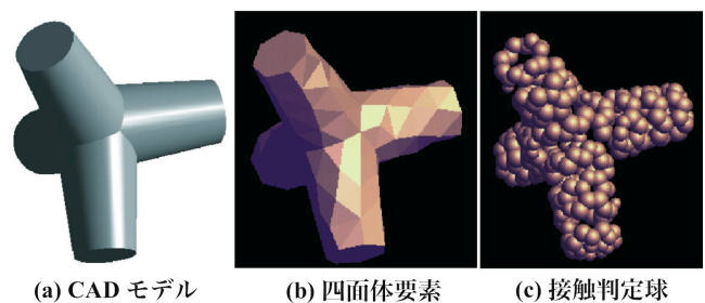
図-5 固体モデル
