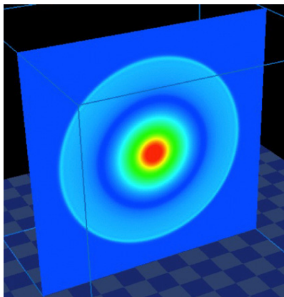
図-2 衝撃波と膨張波の圧力分布 ( t = 0.25 [s])
