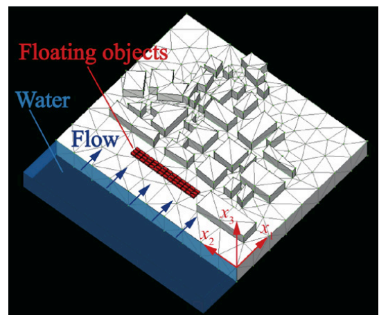
図-8 計算に用いた市街地および漂流物モデル
