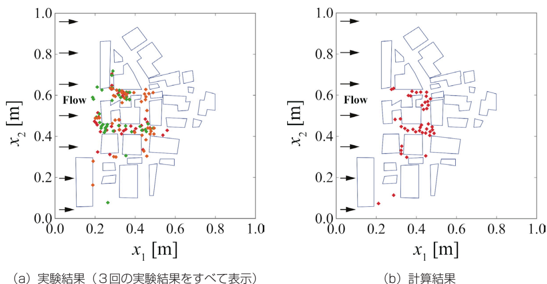
図-10 漂流物の重心点の分布 ( t' = 6.0 [s])
