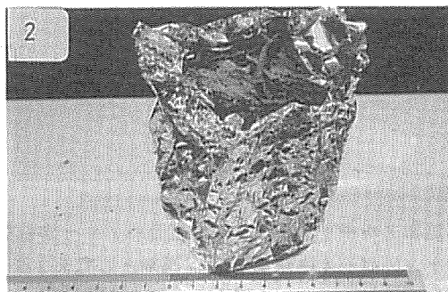
1-2: 風乾後, 土壌サンプルを 40°C で 3 日乾燥させた後, アルミホイルで土壌サンプルを被い土壌の固化剤 (P-レジン) を流しこむ。
