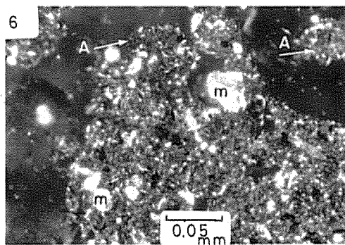
3-6: 団粒の拡大, アモルファス (A) と鉾物 (m) がまじり合って団粒を形成している。
