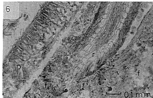
4-6: 落葉 (p) ー分解産物の堆積 (f) からなる積層構造に見られる細根 (r)
