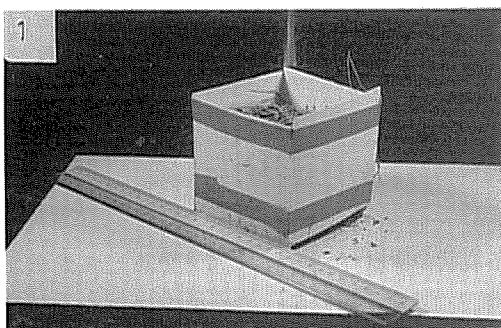
1-1: 10×10 cm のプラスチック板を用いて採集された土壌サンプル。室内において風乾して土壌断面作成の試料とする。
