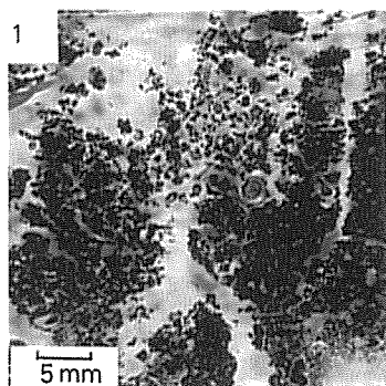
5-1：モダー型でのH層とA 1 層。
