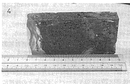
1—4：岩石切断機により作成された土壌サンプル。
