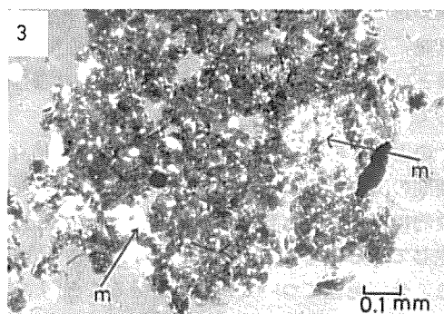
5-3：H層とA 1 層の境界付近の団粒，内部に鉱物(m)がまじっている。
