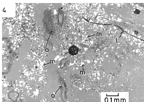
3-4: 偏光下での土壤団粒。白色の部分は、鉾物 (m), 黒色部は有機物 (o), 葉 (l)。
