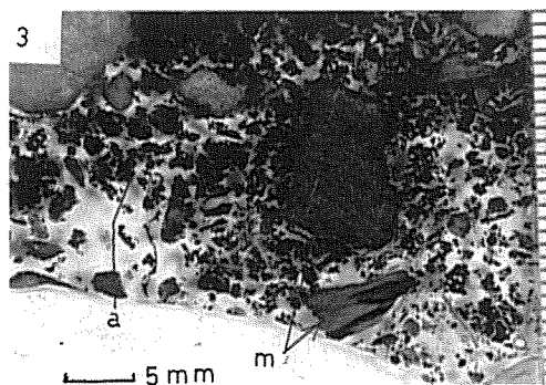
3-3: A 1 層における団粒の分布, 鉾物 (m), 団粒 (a)
