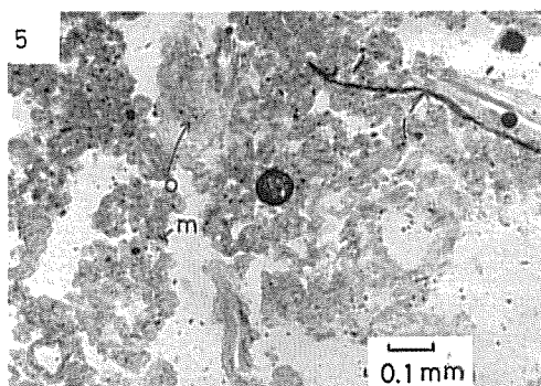
3-5: 3-4と同じ, A 1 層の団粒, 小型のアモルファスの集合に鉾物 (m), 葉 (l), 植物体 (o) が混合している。
