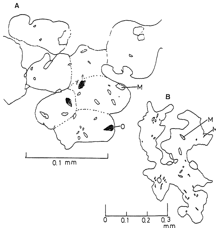
図2 小型の団粒(B)の内部にアモルファス物質と鉱物(M)が交り合っている。団粒をさらに拡大すると、団粒がアモルファス物質を単位としていることがわかる。図Aには8個の単位が示されている。アモルファス単位は鉱物(M)をまじえて、集合している。アモルファス単位内にも鉱物質が認められる。
