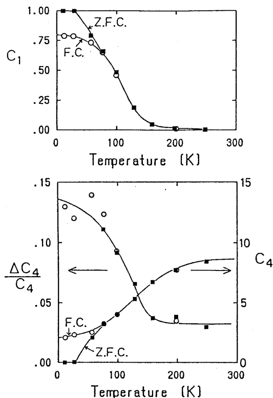
図3 中性子偏極率の波長依存性をフィッティングして得られたパラメータ C_1 , C_4 , \Delta C_4/C_4 の温度変化
