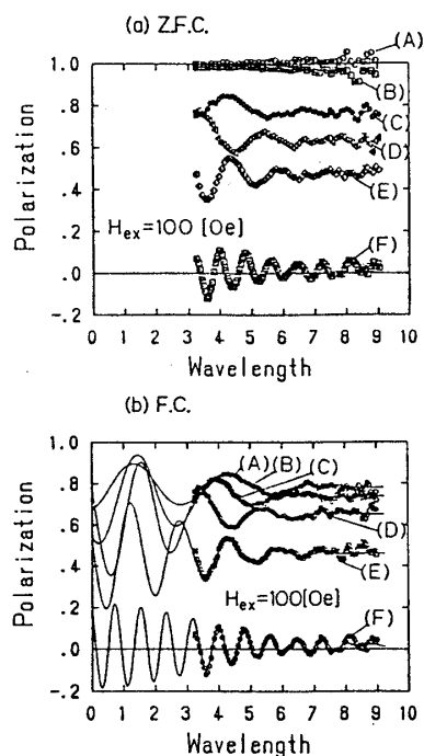
図2 円板状の \text{Fe}_{0.7}\text{Al}_{0.3} (厚さ 0.45 mm) を透過後の中性子偏極度の中性子波長依存性が上記した (A)–(F) の温度に対して示されている。(a) Z.F.C. の場合は、試料を零磁場で 14 K まで冷却した後 100 Oe の外磁場を加えて温度を上昇させ測定した。(b) F.C. の場合は外磁場 100 Oe を加えたまま室温から温度を下降させて測定した。
