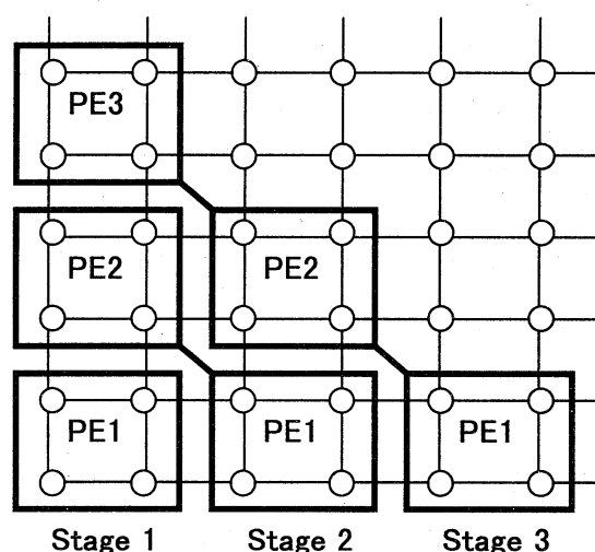
図 2 Block Hyperplane 法
