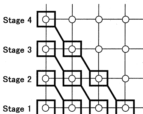
図 1 Hyperplane 法
