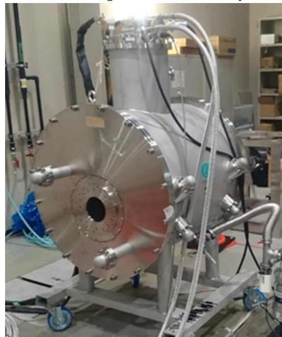
Fig. 1. 3T HTS-MRI magnet.
