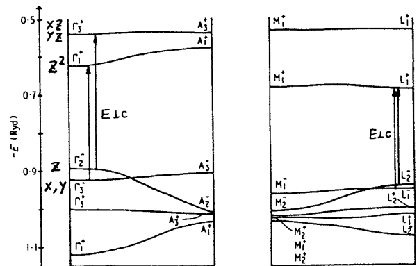
第6図. Murray 1) により計算された, \text{FeS}_2 の電子帯の \Gamma -A, M-L 分散。
