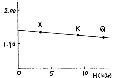
図2. g-値の磁場依存性
