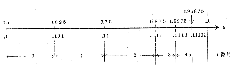
図2-2 ミニマックス有理式近似(2.4)式のため u の [0.5, 1.0) 区間をサブ区分にわけ。
