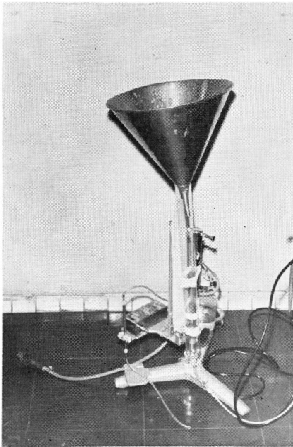
Fig. 2 排尿流率測定装置
