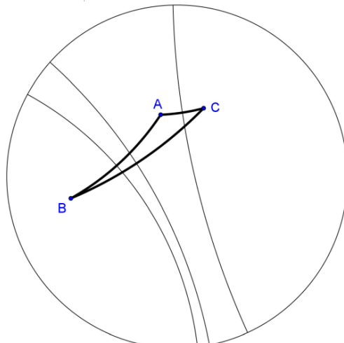
図 14 垂直二等分線が交わらない場合
