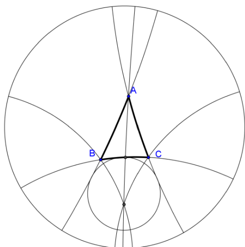
図 17 外角の二等分線が交わる場合
