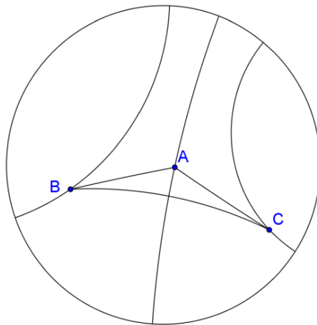
図 16 3 垂線が交わらない場合
