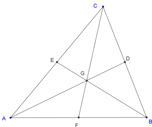
図 10 ユークリッド幾何学における重心
