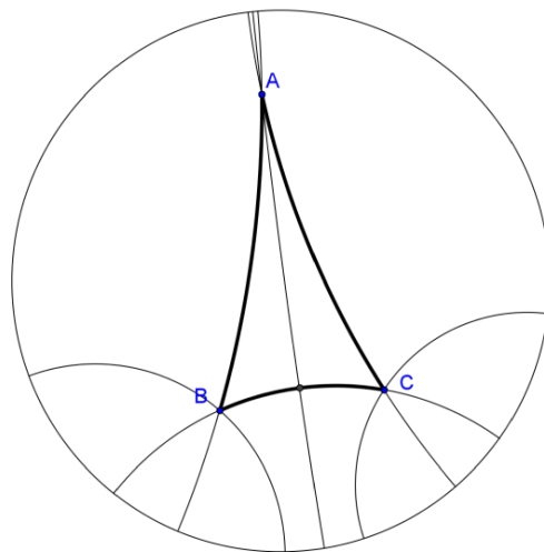
図 18 外角の二等分線が交わらない場合
