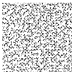
図 3-2：粉の量 c に対するパタンの変化.
