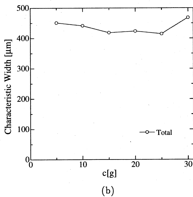
図 4-3：粉の量 c と迷路の幅. (a) 空気の領域 (通路) の幅と粉体領域 (壁) の幅。
