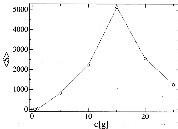
図 4-2：粉の量 c と平均クラスターサイズ S(c) との関係.
