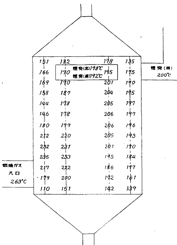
第四圖 有機硫黄除去爐の加熱狀態
