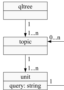
図 4 QueryLogTree のスキーマ
