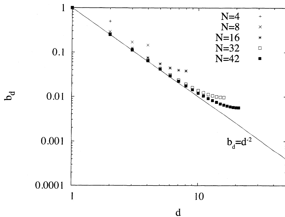
図 1: 結合強度 b_d と格子間距離 d の関係
