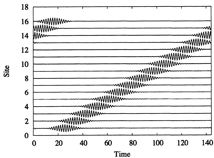
図 3: 対称格子における移動形 ILM の例
