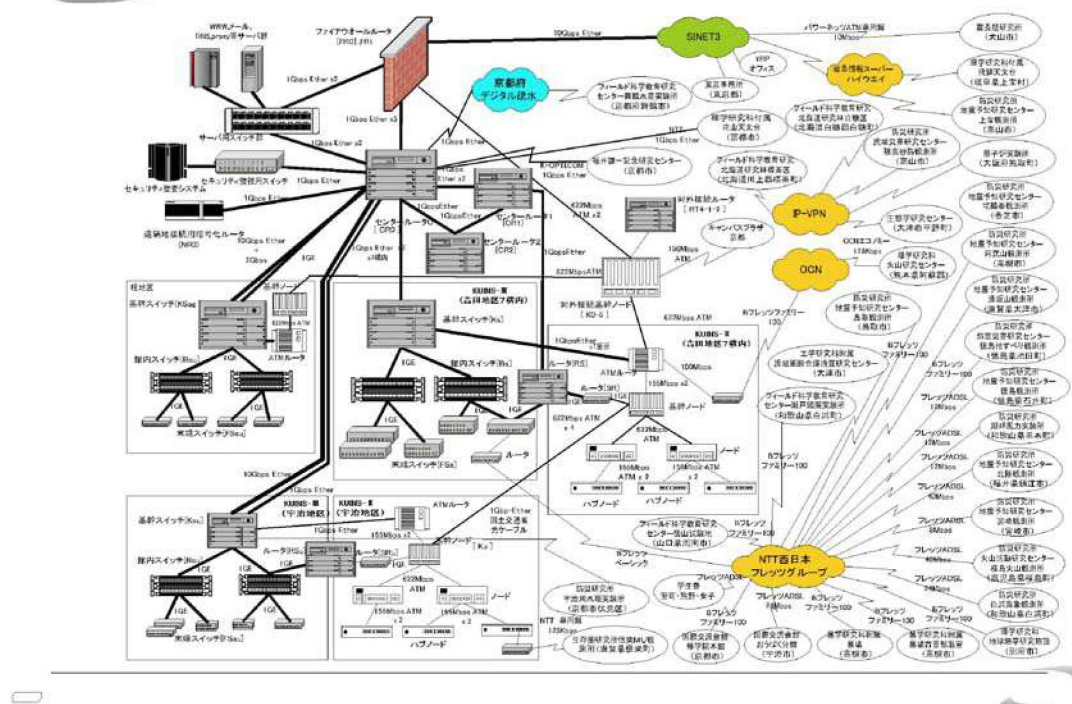
図 1.1.1: ネットワーク構成図 (2008 年 2 月)
