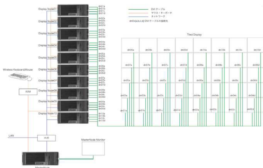
図 0.6.10: タイルディスプレイ構成図
