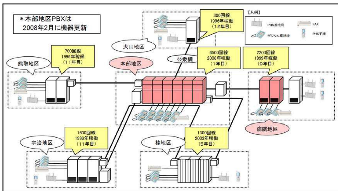
図 1.13.1: 京都大学全体の現行音声ネットワーク図
