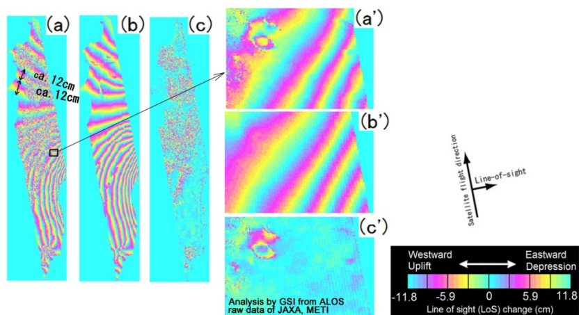
図 1 地殻変動性の長波長成分を除去した SAR 干渉画像
