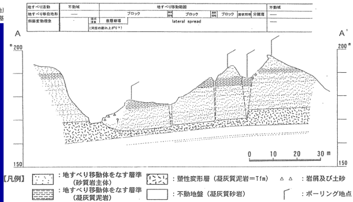
図8 三田盆地西畑のスプレッドの地質断面図 (加藤ほか, 1999)
