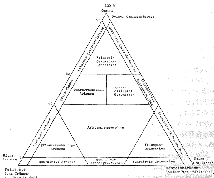
第 8 図 Рухин (1956) による砂岩の分類
