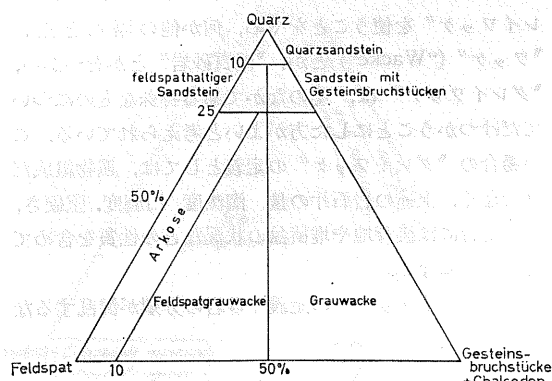
第11図 FÜCHTBAUER (1959) による砂岩の命名図
