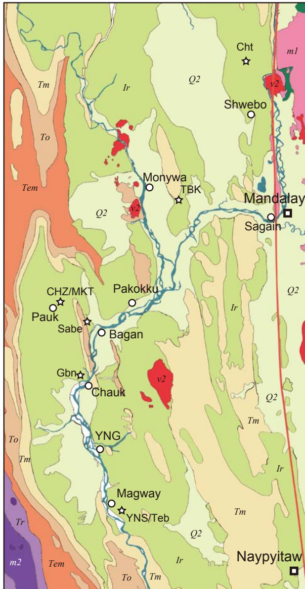
図5. ミャンマー中央部の地質概略図と主な化石産出地点。地名・産地名は表2を参照のこと。地質図はMyanmar Geosciences Society (2014)を簡略化した。Q2, 完新統; Ir, イラワジ堆積層; Tm, ベグー層群上部(またはその相当層, 中新統); To, ベグー層群下部(またはその相当層, 漸新統); Tem, パウンジー層 Paunggyi Formation (モラッセ型堆積物, 晩新統~始新統); Tr, タンバヤ層 Thanbaya Formation (三畳系); m1, 古生代変成岩(一部ジュラ系); m2, 中生代変成岩(主に三畳系); v2, 新生代火山岩。右側の赤太線はザガイン断層 Sagaing Faultを示す。
