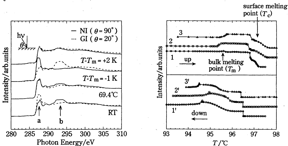
図3 \sigma^*(\text{C-H}) ピークの強度変化
