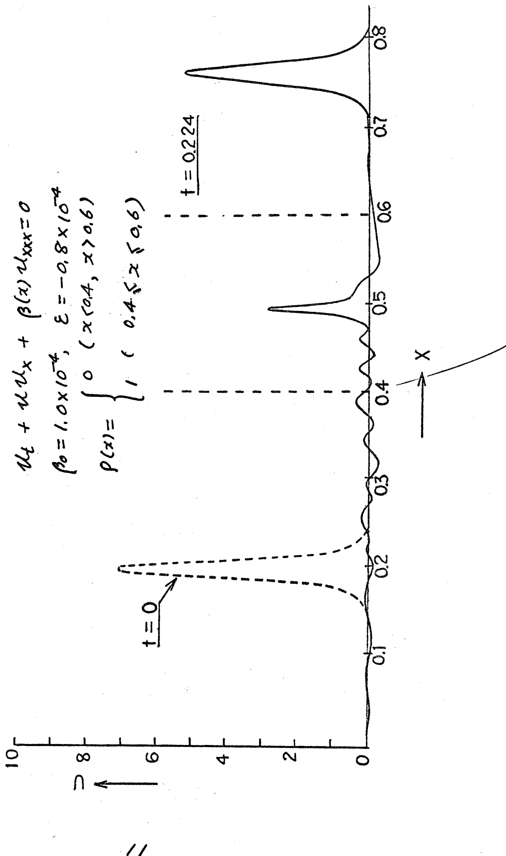
Fig. 1 ソリトンの発生
