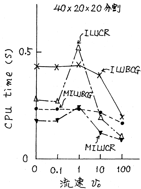
図3.6 S-810での計算時間(風上差分)
