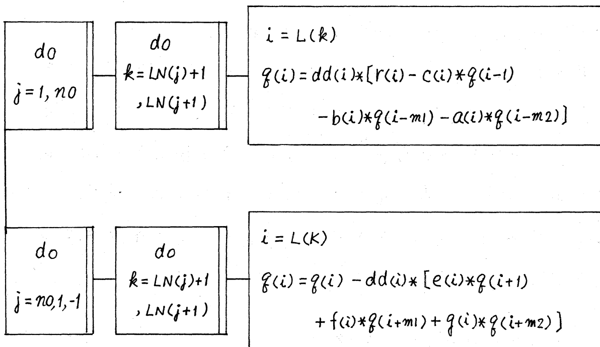
図 2.9 ベクトル計算機向き g = [LDU]^{-1} r の計算
