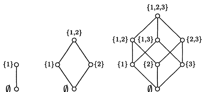
図 1. Boolean 代数
