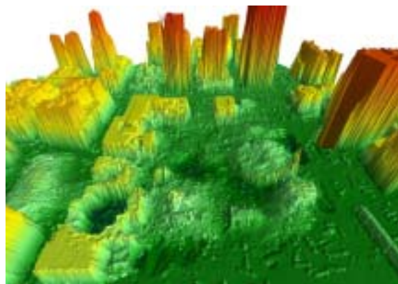
Fig. 6: LIDAR
