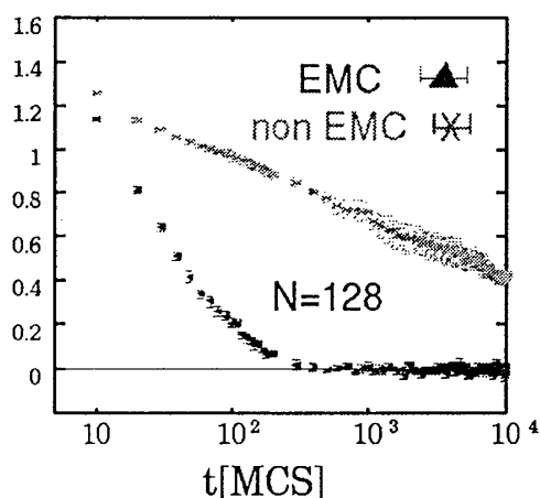
図 2: 2つの異なる定義でのエネルギーの差のモンテカルロステップ依存性。[6] 平衡状態ではゼロになる。上が通常の方法、下が交換法による結果を示す。
