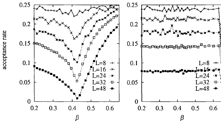
図 1: 交換法における交換確率を逆温度の関数として示す。左は逆温度を等間隔で設定したもの、右は文献[2]の方法で設定した温度を用いた。どちらも最低温度と最高温度、全温度数は等しい。
