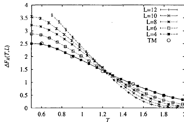
図 3: 3次元 \pm J Ising スピングラス模型の自由エネルギー差の温度依存性。転移温度 ( T_c \sim 1.1 ) を境に、サイズとともに減少する高温相と増加するスピングラス相の違いがよくわかる。
