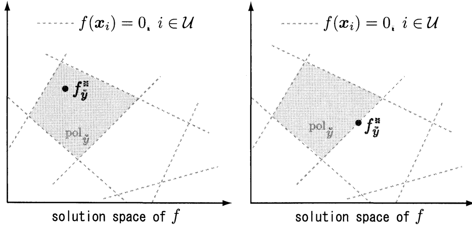
図 2: 条件付最適解 f_y^* と局所最適解の関係: (左) 条件付最適解 f_y^* が凸ポリトープ \text{pol}_y の内点である場合は S^3\text{VM} の局所最適解となるが, (右) 条件付最適解 f_y^* が凸ポリトープ \text{pol}_y の境界上にある場合は S^3\text{VM} の局所最適解とはならない.
