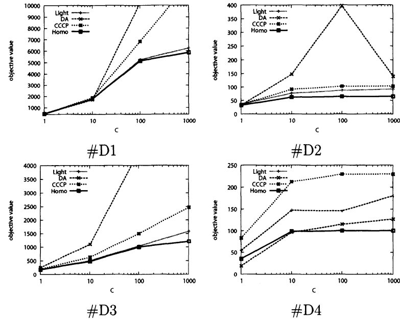
図 3: 各アルゴリズムの最適化性能の比較
