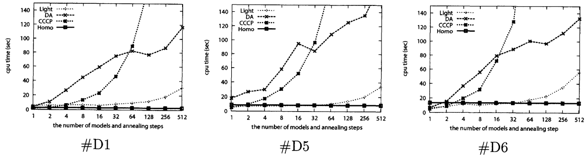
図 4: モデル選択における計算コスト
