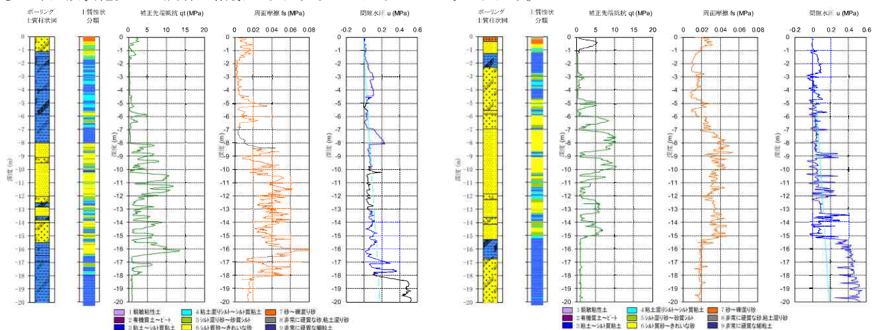
(地点1) (地点3) 図-1 CPTのプロファイル
