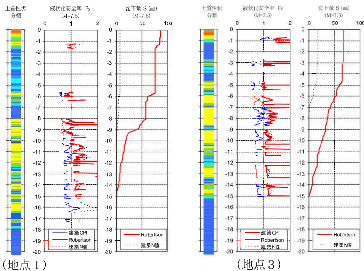
図-7 FI法による液状化判定結果および地盤沈下量の推定 (M=7.5, \alpha=1.5\text{m/s}^2 )
