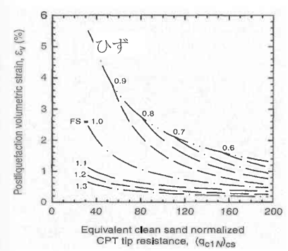
図-5 等価クリーンサンド先端抵抗と体積ひずみとの関係
