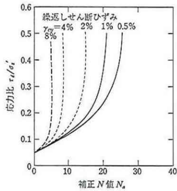
図-4 補正N値と繰返しせん断ひずみとの関係
