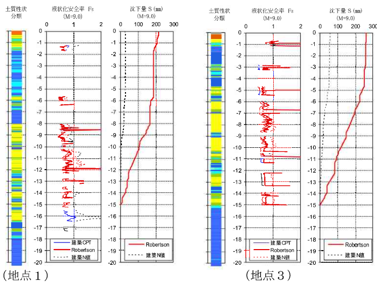
図-6 FI法による液状化判定結果および地盤沈下量の推定 (M=9.0, \alpha=1.5\text{m/s}^2 )
