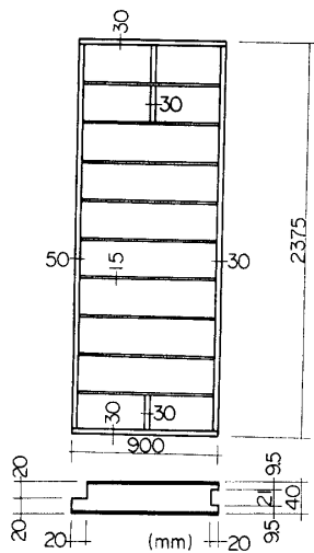
図6 試験体図 No. W-7, 11, 15 図7 試験体図 No. W-8, 16 図8 試験体図 No. W-9, 17(mm)
