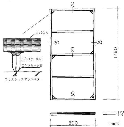
図16 試験体図 No. F-23
