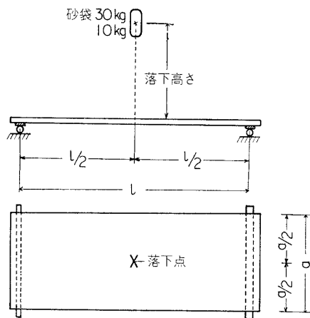
図36 衝撃荷重試験・砂袋落下式 壁パネル l=2200 mm
