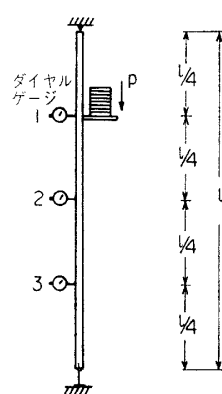
図27 面に平行な積載荷重試験
