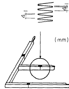
図14 No. W-30 のコア横 におけるフィンガー ジョイント (パネルの構成は図13に 同じ)
