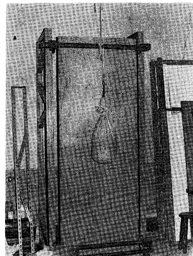
写真6 衝撃荷重試験・砂袋振り式
