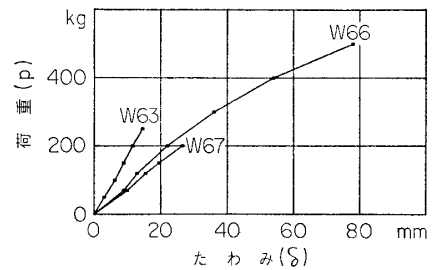
図37 壁パネルの面に垂直な積載荷重試験の荷重—たわみ曲線，図中の番号は試験体 No.
