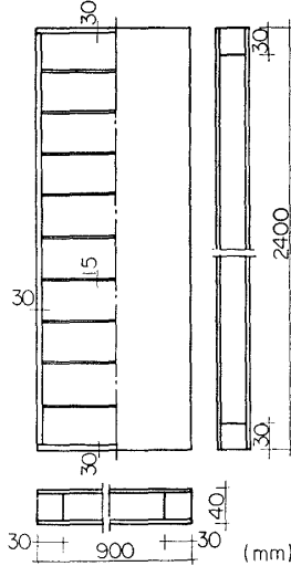
図13 試験体図 No. W-29
