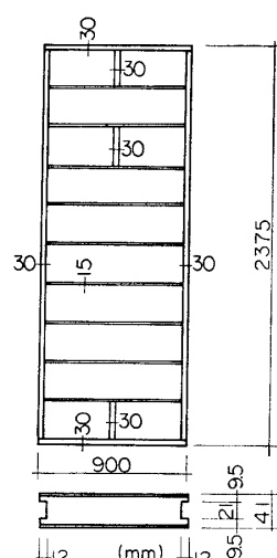
図6 試験体図 No. W-7, 11, 15 図7 試験体図 No. W-8, 16 図8 試験体図 No. W-9, 17(mm)
