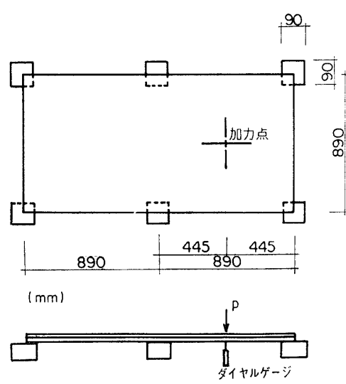
図30 局部荷重試験・試験体 No. F-24
