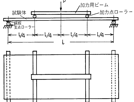
図21 面に垂直な積載荷重試験 壁パネル l=2200 mm 床パネル l=1700 mm
