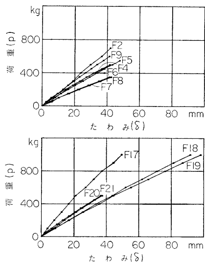
図39 壁パネルの局部荷重試験の荷重—たわみ曲線，図中の番号は試験体 No
