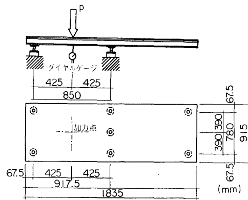
図34 局部荷重試験・試験体 No. F-29
