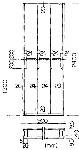
図9 試験体図 No. W-25 堅柱，中堅横たて継(突付)そえ木接着
