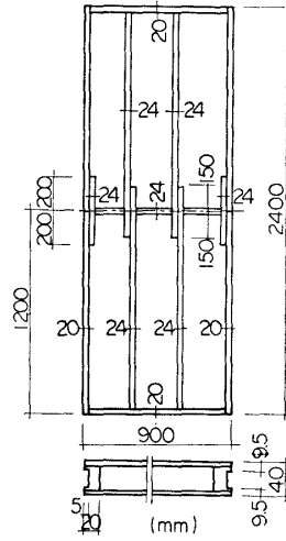
図10 試験体図 No. W-26 中堅横ラップジョイント(接着)
