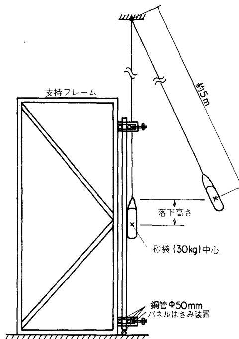
図35 衝撃荷重試験・砂袋振子式
