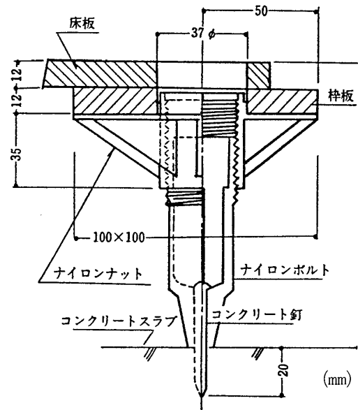
図19 試験体 No. F-25, 26 に使用したプラスチックジャスター詳細図
