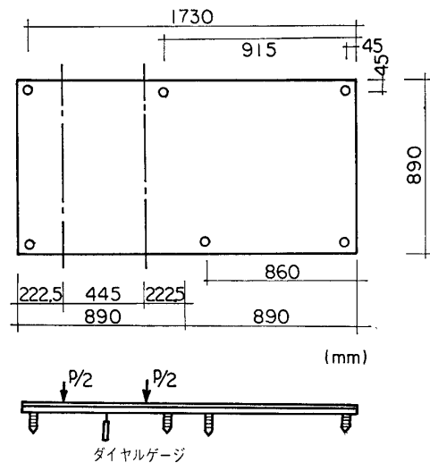
図23 面に垂直な積載荷重試験・ 試験体 No. F-23
