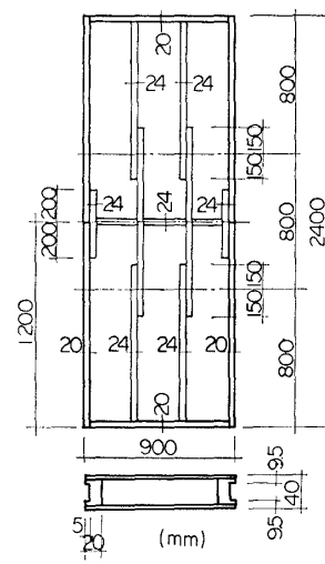
図11 試験体図 No. W-27
