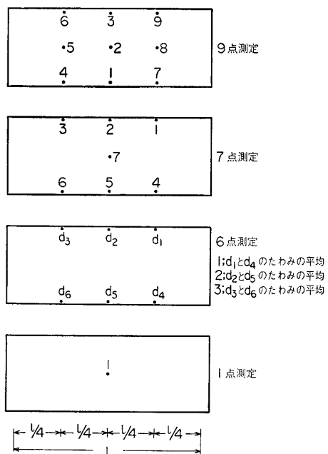
図22 たわみ測定点 図中 1～9 の番号は付表で使用した測点番号
