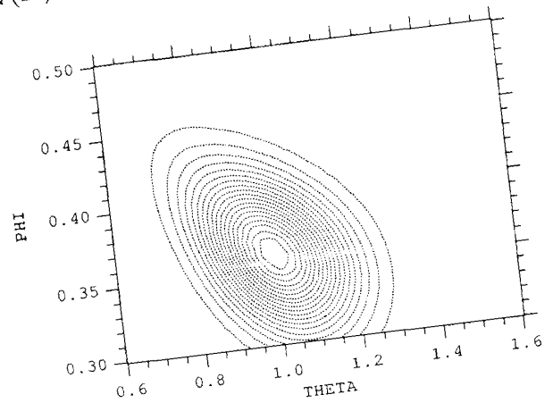
図 6. 状態数密度 \Lambda(\phi, \theta)
