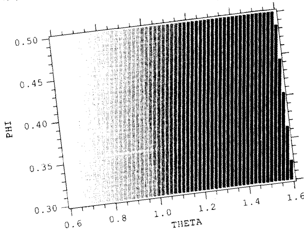
図 5. ポテンシャルエネルギー V(\phi, \theta)
