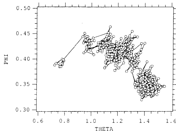
図4. \phi - \theta 平面上の軌跡
