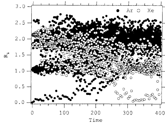
図 2. R_i の時間変化
