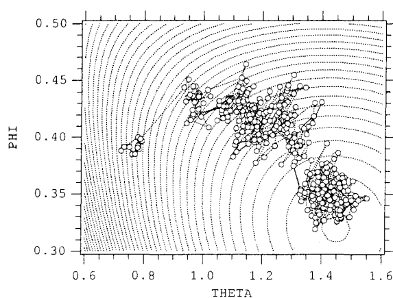
図 8. エントロピー S(\phi, \theta)
