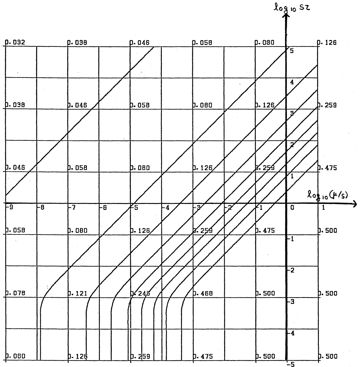
第5図. 擾動淘汰様式の平均ヘテロ接合度 \langle H \rangle への影響 ( \delta = \frac{1}{2} とおいた淘汰様式(5.1)の下での拡散過程モデル(5.5)による \langle H \rangle ). s = 10^3 と固定した, \mu × s 平面 ( \log_{10}(\mu/s) , \log_{10} sz ) 上の等高線図)
