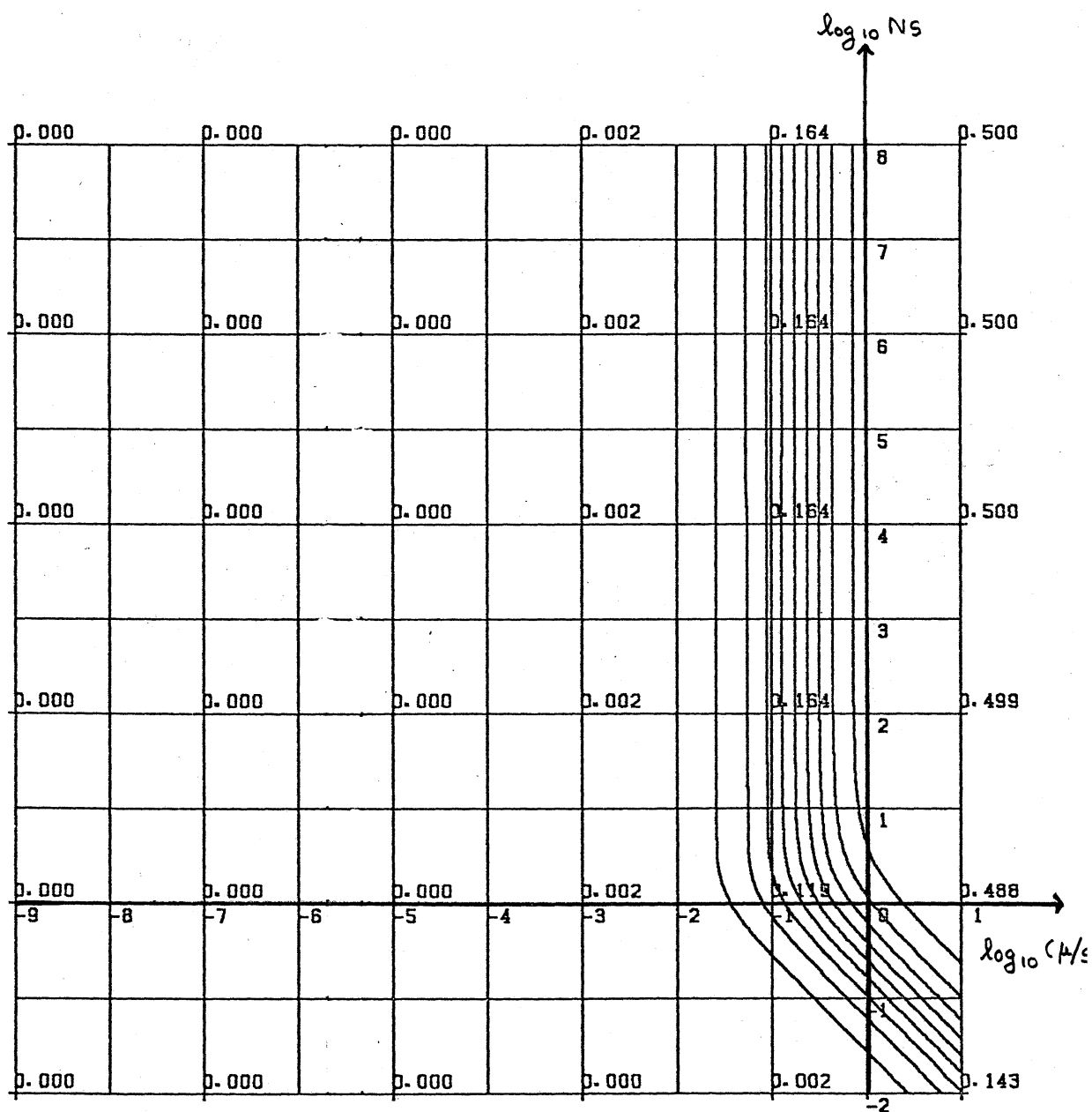
第3図. サイズ効果の下での平均ヘテロ接合度 \langle H \rangle (拡散過程モデル(4.1)による. パラメタ平面 (\log_{10}(\mu/s), \log_{10} Ns) 上の等高線図)
