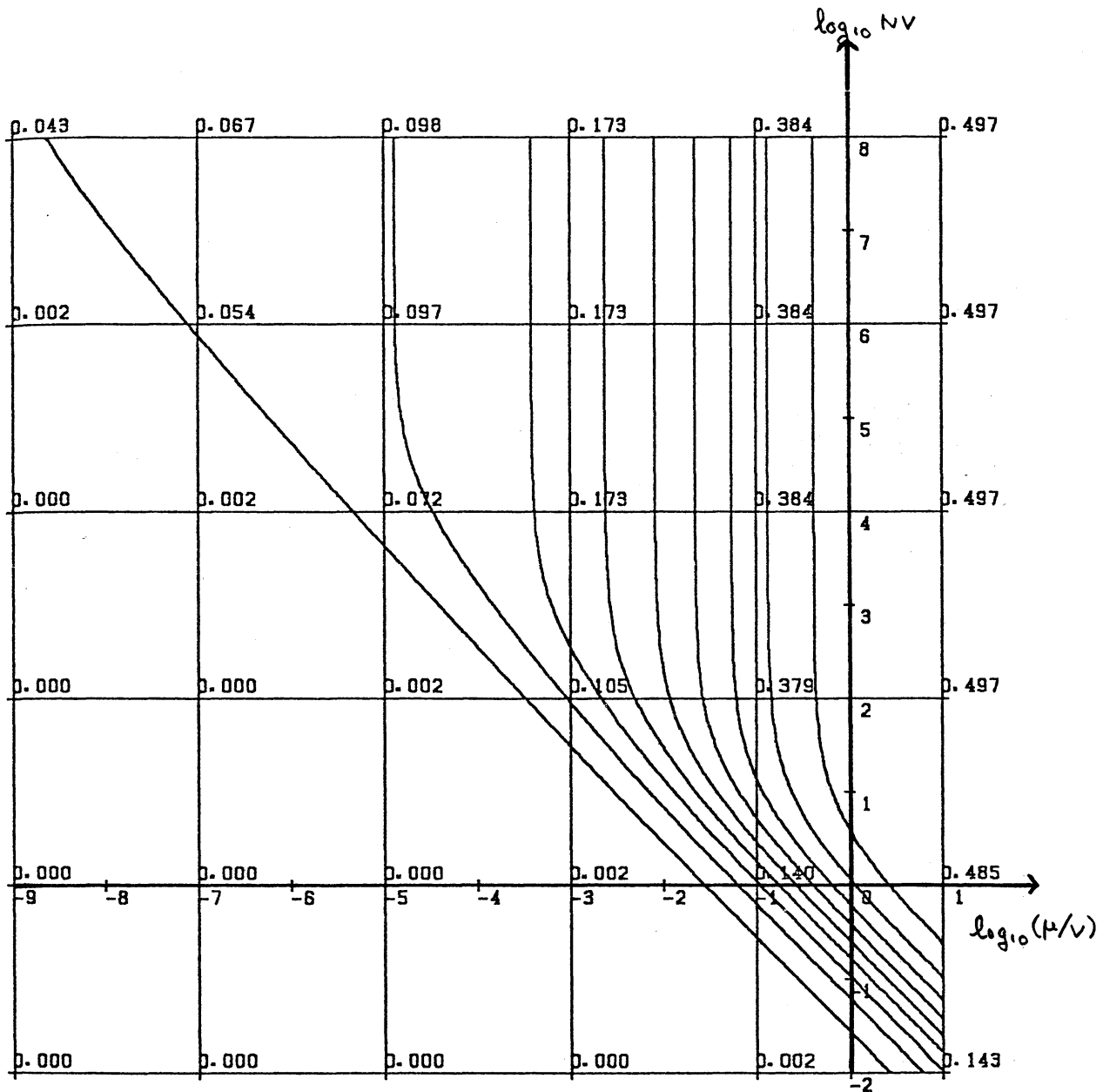
第4図。揺動淘汰とサイズ効果の下での平均ヘテロ接合度 \langle H \rangle (拡散過程モデル(4.3), (4.4)による, \log_{10} NV 平面( \log_{10} (\mu/v) , \log_{10} NV )上の等高線図)
