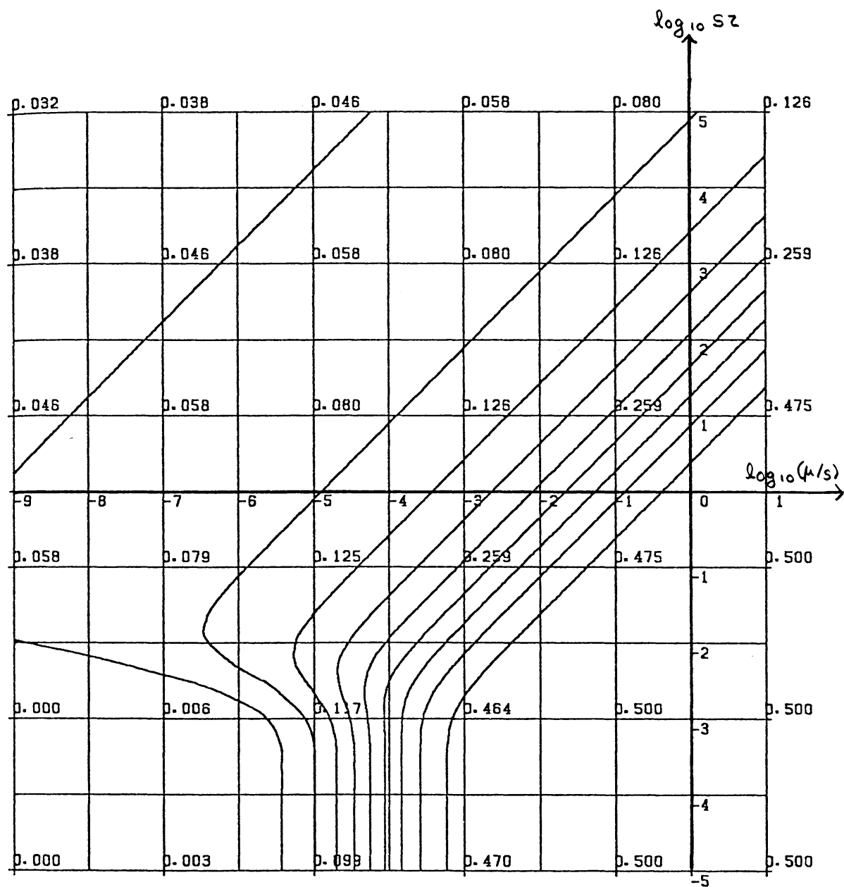
第2図. 拡散過程モデル(3.16)~(3.18)の平均ヘテロ接合度 \langle H \rangle ( s = 10^3 を固定した, \log_{10}(\mu/s) 平面 ( \log_{10}(\mu/s) , \log_{10} sz ) 上の等高線図)
