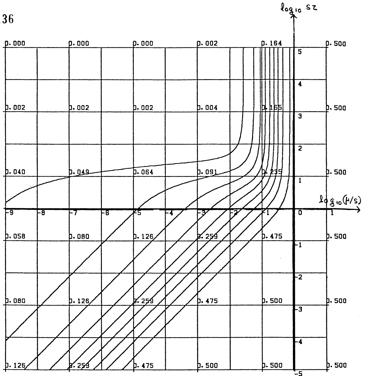
第1図. 確率力学系モデル (3.14), (3.15) の平均ヘテロ接合度 \langle H \rangle (パラメータ平面 (\log_{10}(\mu/s), \log_{10} s^2) 上の等高線図)
