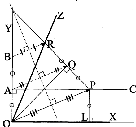
図 3.1: 角の三等分
