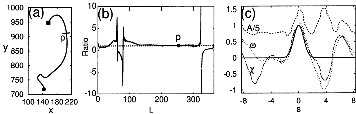
図5: 典型的な T 渦構造 (a) スケルトン (●: 始点、■: 終点) 座標はメッシュサイズが単位。(b) スケルトンに沿っての、 \chi と \omega の比。バーガス T 渦解が1になるように規格化している。(c) p点をよぎる垂線上の \chi(s) 、 \omega(s) 、 A(s)/5 。 \chi と \omega は p 点上で1になるように規格化してある。実線はガウシアン。
