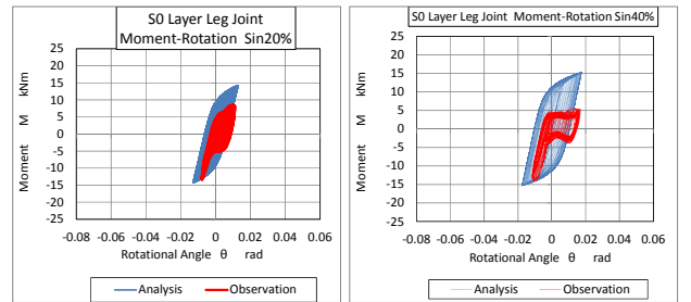
a) 20% sin wave input
