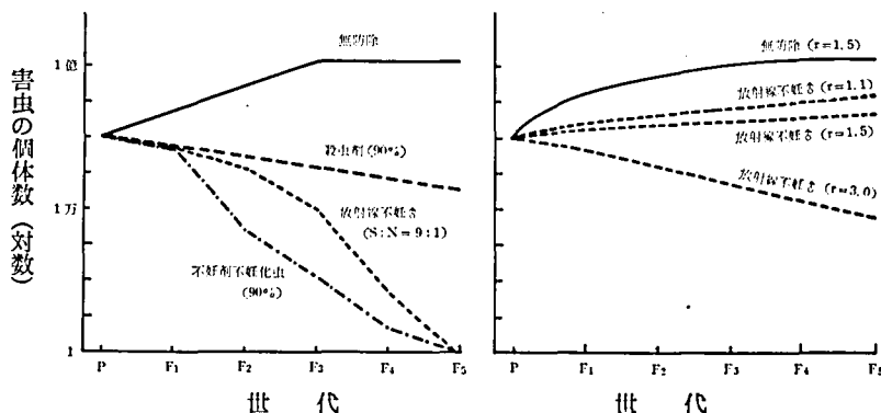
第7図 左. 害虫個体群に対する殺虫剤 (90%の防除効率), 放射線不妊化雄放飼 (最初の世代の野生雄個体数 (N) に対して9倍の不妊化雄 (S) を毎世代放飼する) 及び不妊剤による不妊化 (90%不妊化) 法の影響。但し、飽和密度1億2千5百万頭に至るまでは毎世代5倍ずつ増殖する。性比は1:1 Knippling (1964) 64) を作図。
