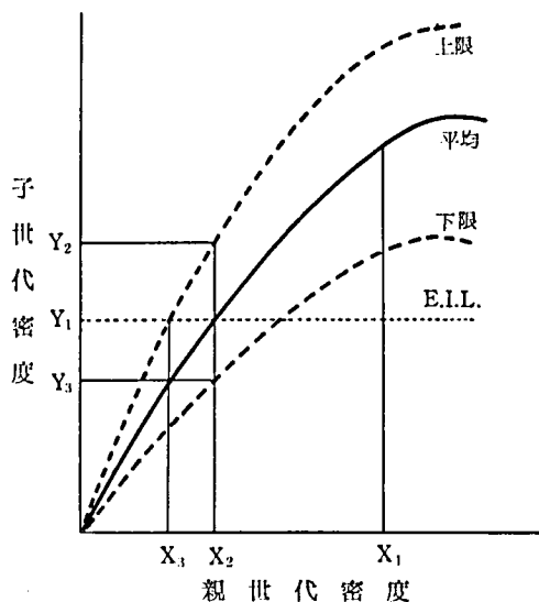
第3図 不確定要因が働かない場合(実線)と働く場合(点線)の増殖曲線からみた要防除密度。当世代は被害を与えないが次世代にはE.I.L.以上に密度が増えると被害が出る。X 1 は現在の害虫密度、X 2 は、次世代に被害がみられる密度。Y 1 , Y 2 は不確定要因が働く時の次世代に被害が出る最少密度と最高密度をそれぞれ示す。
