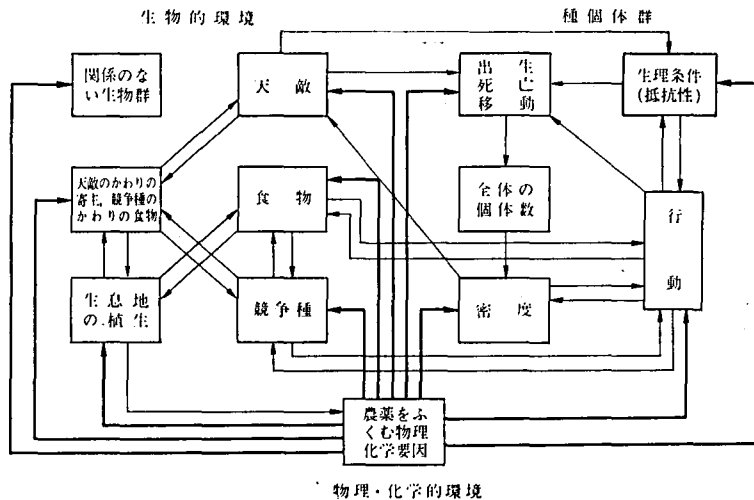
第1図 SOLOMON 100) が示した種の生活系 (life system) の構造。ここでは農薬が生活系にもたらす直接的影響 (太線) と間接的影響 (細線) をとりあげた。
