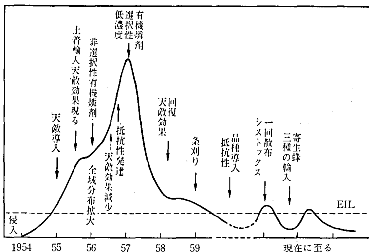
第10図 カルフォルニア州におけるアルファルファブラムシの防除経過
