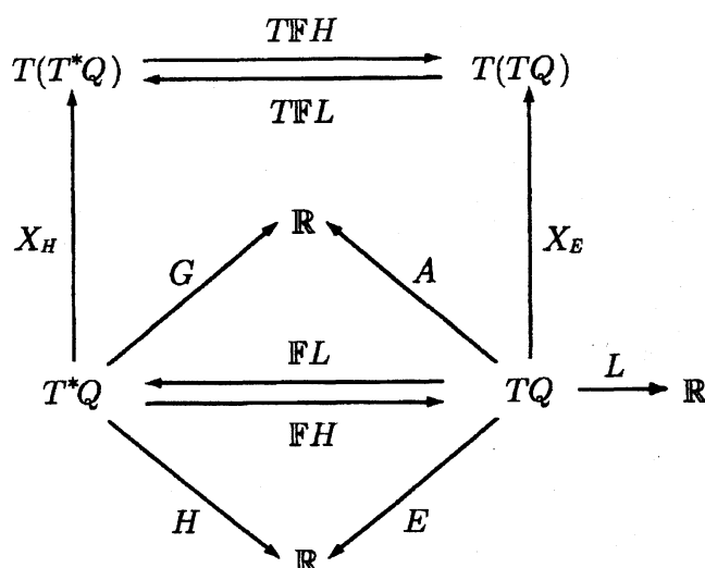
図 1: ラグランジアン系とハミルトニアン系の基本構造
