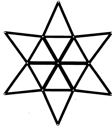
図 2: 24 部材球形シェル状トラスの最適解
