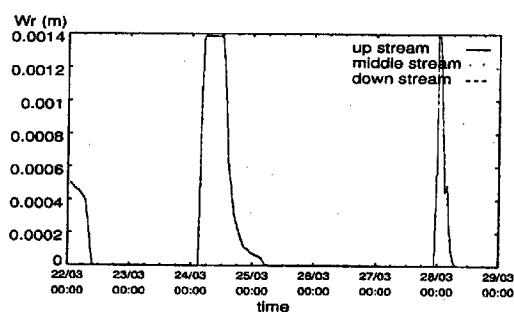
Fig. 10 貯留水分量
