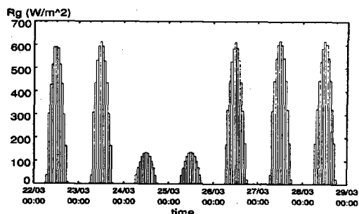
Fig. 3 全天日射量
