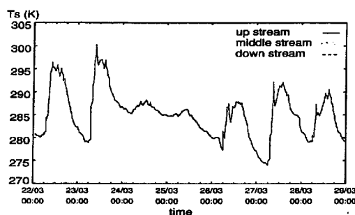
Fig. 8 表面温度
