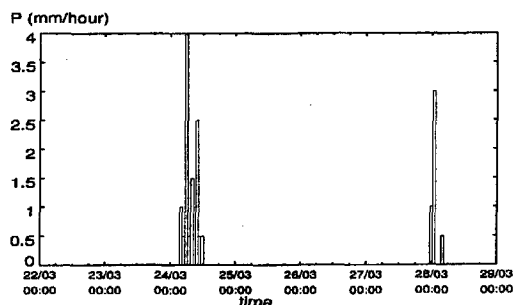
Fig. 2 降雨量
