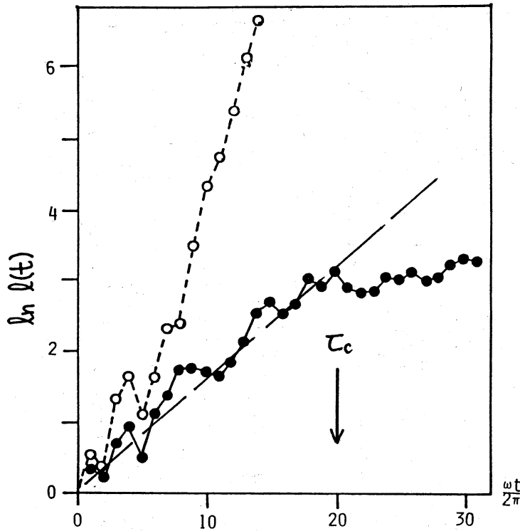
Fig. 4 DRM の等高線の長さ l(t) の時間変化。破線は古典論で実線は量子論。パラメーターの値は Fig. 3 と同じである。これから \alpha_1 \sim 0.60 , \alpha_2 \sim 0.17 , \tau_c \sim 20 を得る。
