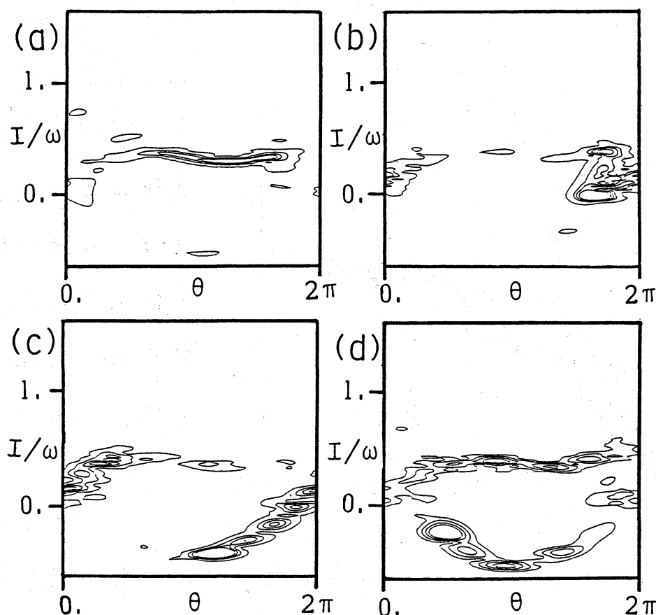
Fig. 3 DRMの量子論で分布関数の示す heteroclinic構造におけるうなりの発生
