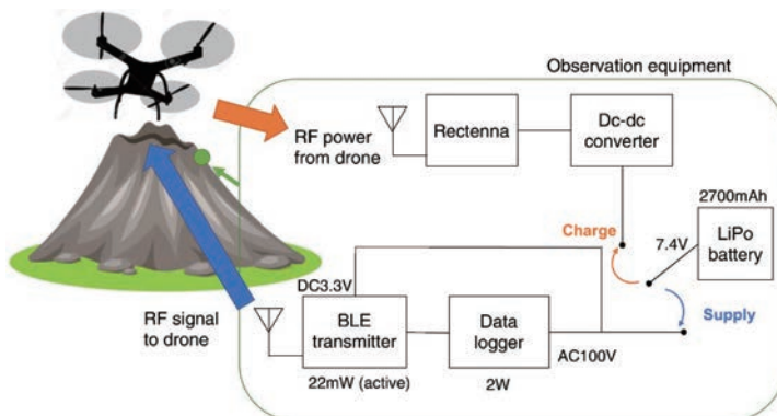
図1：提案するドローンを用いたマイクロ波送電システム
