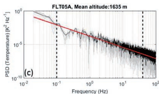
図1：高度1635mのUAV水平飛行で得られた気温の周波数スペクトル。赤線は傾き -5/3 乗を示す。[Luce et al., 2019]
