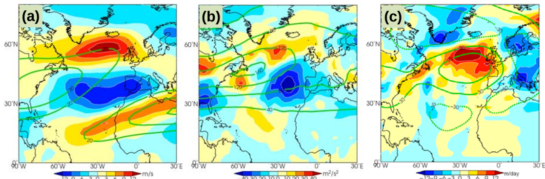
図 10 2011/2012 年冬平均 (a) 300hPa 東西風速平年偏差、(b) 300hPa 高周波擾乱の運動エネルギー平年偏差、及び (c) 高周波擾乱による渦度フラックスの収束に伴う 300hPa 高度変化率 (m/day) 平年偏差 等値線は、(a) 平年値を示し西風 20m/s 以上を 10m/s 間隔で表示、(b) 平年値を示し 40m 2 /s 2 間隔で表示、(c) 300hPa 高度偏差を示し間隔は 30m。高周波擾乱成分は 2～8 日のバンドパスフィルターをかけて求めた。
