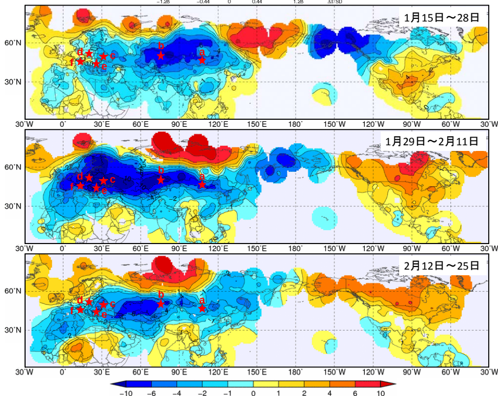
図 2 2012 年 1 月 15 日から 2 月 25 日の 2 週ごとの気温平年差 (°C) 各国から通報データによる。図中の星印 (a～f) は以下の地点 (国名) の位置を示す。
