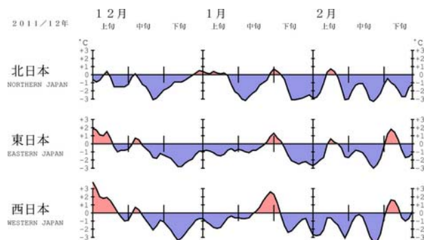
図3 地域平均気温平年差の5日移動平均時系列 (2011年12月～2012年2月)
