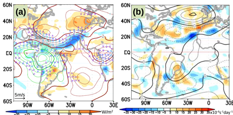
図 12 2011/2012 年冬平均 (a)200hPa 速度ポテンシャル平 年偏差 (等値線)、200hPa 発散 風年偏差 (矢印)、及び外向き 長波放射 (OLR) 年偏差 (陰影)、 (b)200hPa ロスビー波ソース (陰 影) 及び 200hPa 流線関数年偏 差 (等値線) 等値線間隔は (a) 0.5 \times 10^6 \text{ m}^2/\text{s} 、 (b) 3 \times 10^6 \text{ m}^2/\text{s} 。
