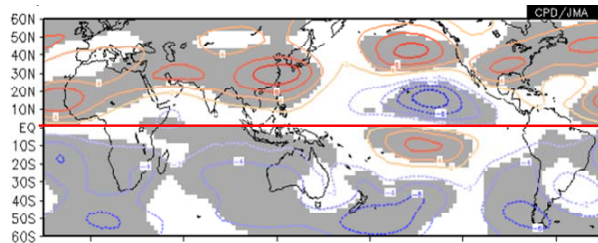
図 11 冬平均 200hPa 流線関数平年偏差のラニーニャ年の合成図
