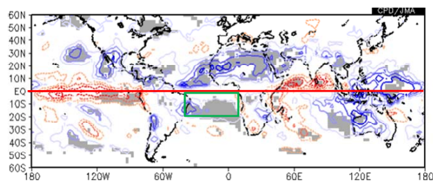
図 13 南大西洋熱帯域 (20°S~赤道、40°W~10°E) で 領域平均した冬平均海面水温に対する冬平均外向き長 波放射 (OLR) の回帰係数
