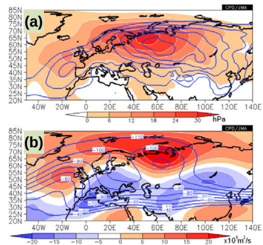
図7 2012 年 1 月 16 日～2 月 14 日平均 (a) 海面気圧、(b) 300hPa 流線関数 陰影は年間偏差。等値線は (a) 1020hPa 以上を 5hPa 間隔で、(b) -40 \times 10^6 \text{ m}^2/\text{s} 以下を 10 \times 10^6 \text{ m}^2/\text{s} 間隔で表示。
