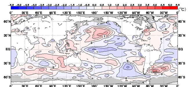
図6 2011/2012 年冬平均海面水温年間偏差
