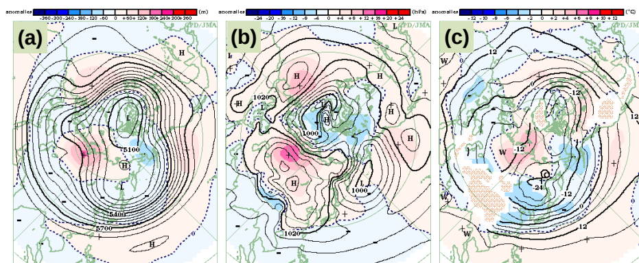
図4 2011/2012年冬平均(a)500hPa高度、(b)海面気圧、及び(c)850hPa気温。等値線間隔は、(a)60m、(b)4hPa、(c)4°C。(c)の波状の陰影域は標高が1,600m以上の領域を示す。
