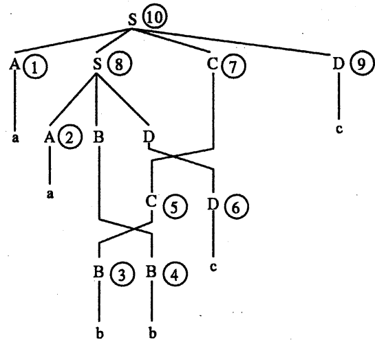
図 4: 入力 I = aabbcc に対する構文解析木
