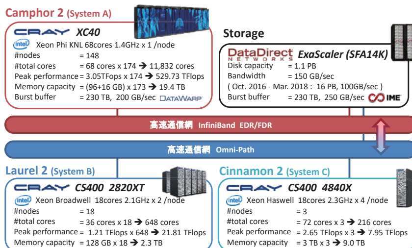
図 1： 電波科学計算機実験装置(KDK)概略図。学術情報メディアセンターと共同調達している。数値は平成 30 年度に KDK として利用可能な資源を示す。総理論演算性能は 559.50 TFlops である。
