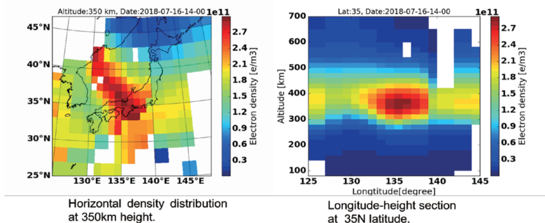
図5 リアルタイムトモグラフィ解析結果の例
