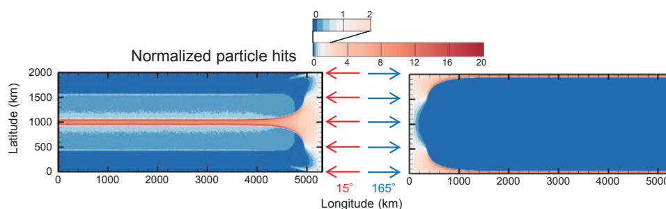
図 3 : 火星南半球の磁場異常地域における地表面の宇宙放射線量分布 (左 : 東側入射 15^\circ 、右 : 西側入射 165^\circ )
