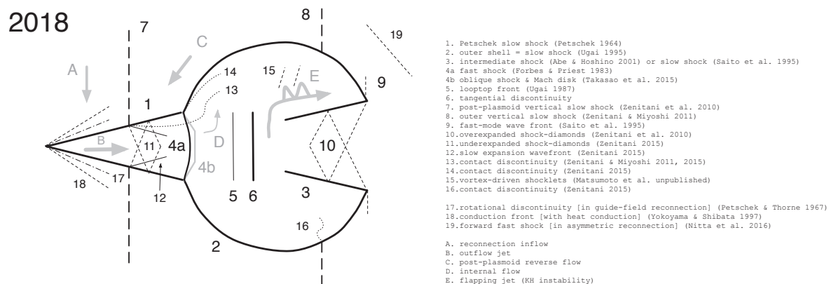
図 1 磁気リコネクションで生成される磁気島（プラズモイド）構造のまとめ図。2018 年版。
