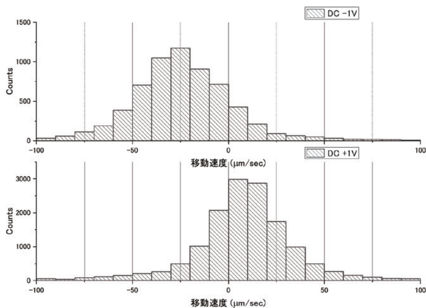
図2 粒子の移動速度の統計解析
