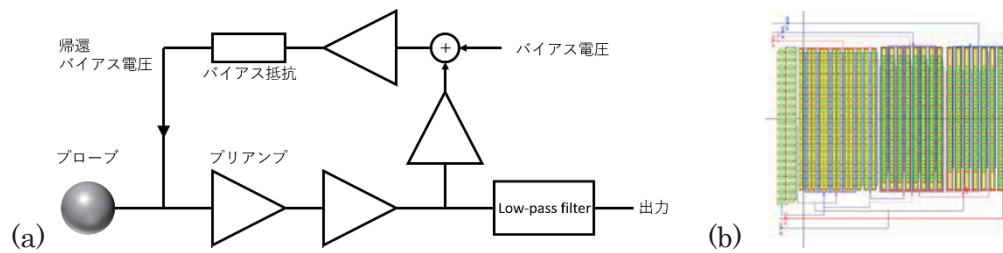
図 1：電場観測用 (a) ブロック図と (b) 基本オペアンプ
