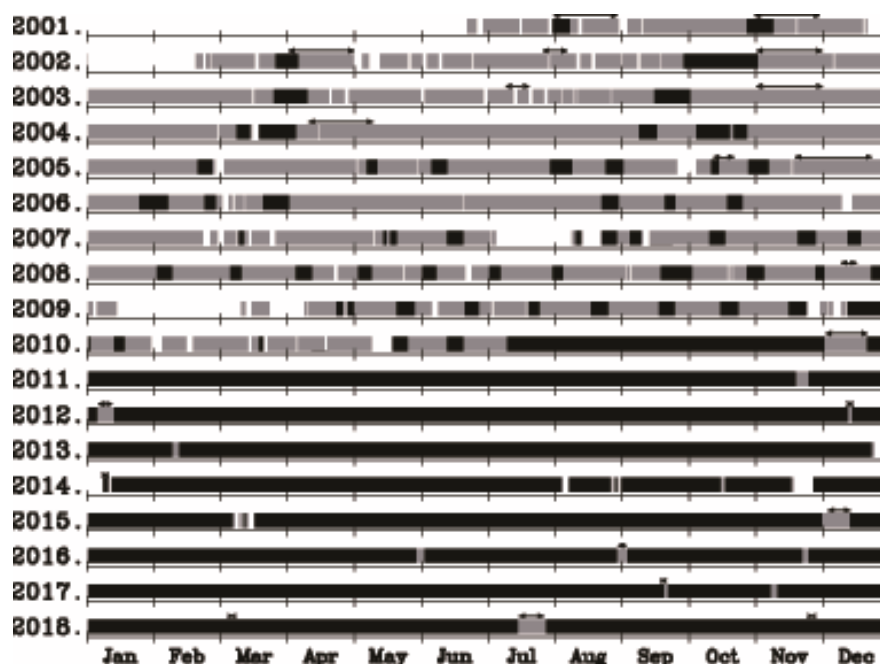
図 5. 赤道大気レーダー長期連続観測の実績（濃色部分：電離圏観測を同時実施）
