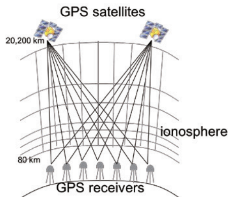
図4 GPS トモグラフィの概念
