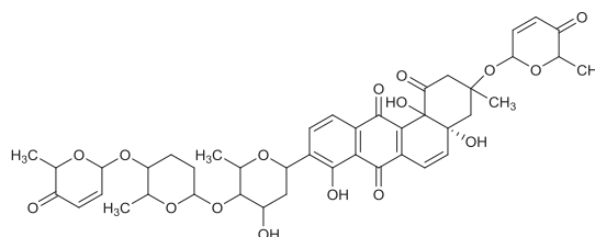
図. 2 サブロルマイシン E の構造
