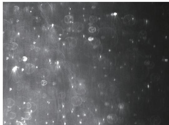
図1 固体粒子(100nm)の撮像
