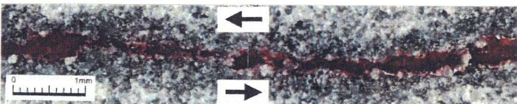
(d) Shear displacement of 1mm
