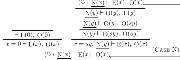
図4 CLKID ω の証明の例
