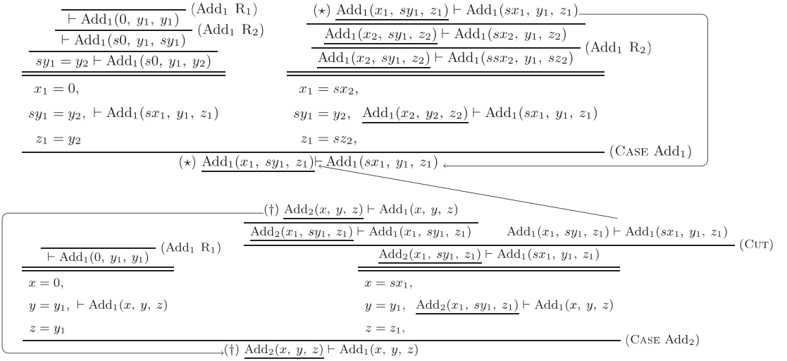
図 6 \text{Add}_2(x, y, z) \vdash \text{Add}_1(x, y, z) に対する \text{CLKID}^\omega の証明
