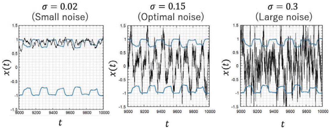
図3 SMG(2) の各ノイズ強度のサンプルパス. 黒線は x(t) の時系列, 青線は決定論アトラクターを表す. パラメーターは a = 0.14, b = 0.1, c = 10, \tau = 90 である.
