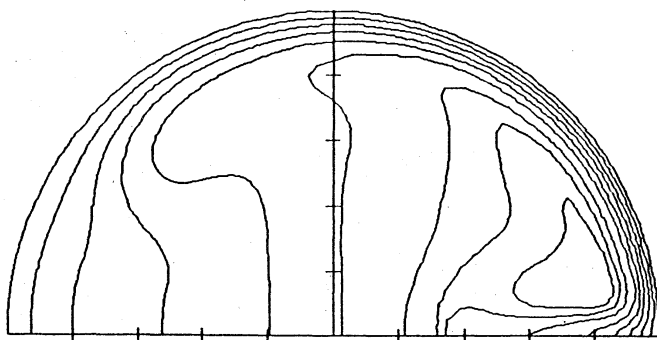
図4. Dn=10000 の流線(上)及び管軸方向等速度線(下)
