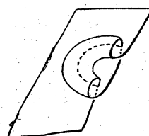
R^+ -disk
