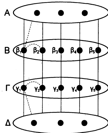
図2 オーダーが5の強 X -type.
