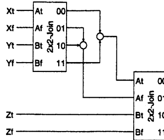
(b) 二段目の 2x2-Join 回路まで設計
