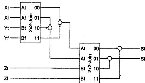
図 8: 全加算器の和 (S) を計算する回路
