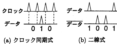
図 1: 回路方式
