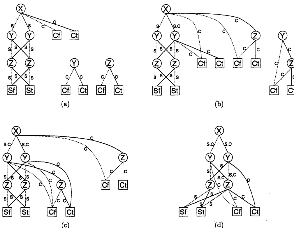
図 10: 全加算器のグラフの作成過程
