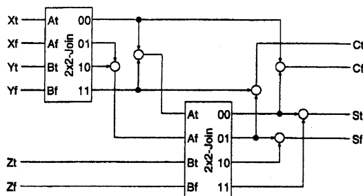
図 13: 全加算器の回路図
