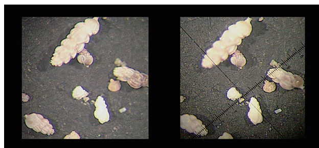
図1 海洋底に生息するブドウのような形の Uvigerina 属（底生有孔虫）のステレオ写真。個体のサイズは約0.3-1mm。立体視できますのでお試しください。
