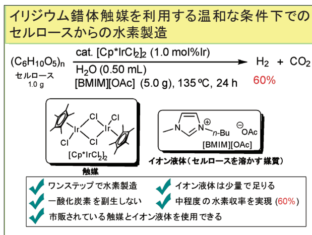
図版13 イリジウム錯体触媒を利用する温和な条件下でのセルロースからの水素製造
