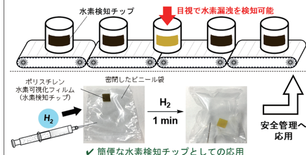
図版 14 見えない水素を検出するための水素検知フィルムチップの開発
