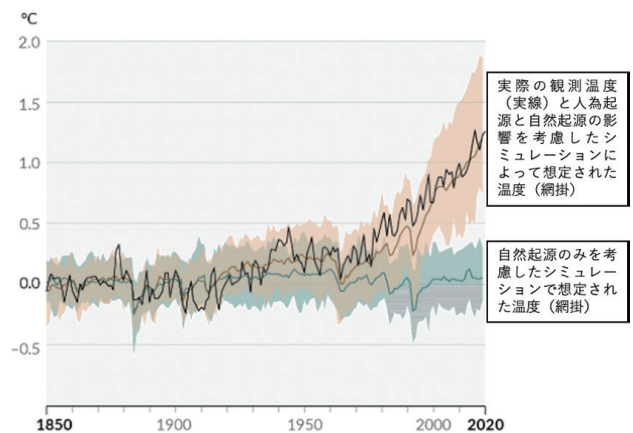
図 4 世界の平均気温の変化（黒実線）と、人為起源要因の有無で分けてシミュレーションした結果。縦軸は 1850-1900 年の平均との差分。いずれの場合も 1940-1970 年代に一時的な気温低下が確認できる（IPCC 第 6 次報告書より）。なお、人間活動に起因する大気中の微粒子の増大と自然に生じる数十年周期の気候の寒冷化が同時期に起きたことも、この時期の気温低下の一因であると指摘されている（Aizawa et al, 2022）。
