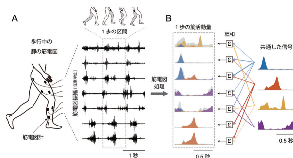
図1 歩行中の脚の筋電図および算出された共通信号 (A) 歩行時(3歩)の脚の筋電図信号。上から、大腿直筋、大殿筋、外側広筋、大腿二頭筋、前脛骨筋、腓腹筋、ヒラメ筋の筋電図を示している。(B) 1歩の筋電図信号を処理して得た筋活動(灰色)がそれぞれ、4つの共通信号(青・赤・黄・紫色)の組み合わせとして表現できることを示す。図は、Hagio et al., 2015 をもとに作成。
