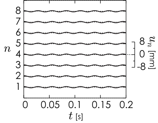
(d) No ILM
