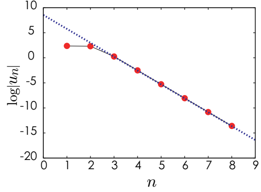
(b) P1-2( T = 3.75139 )
